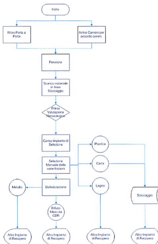
Figura 5 - Schema del processo di recupero carta e plastica
