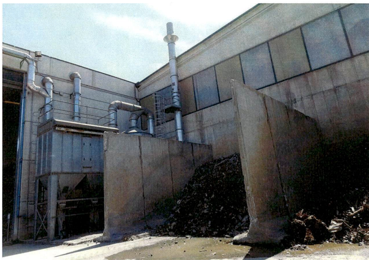
Figura 10-6 – Emissione E2 e stoccaggio rifiuti prodotti
